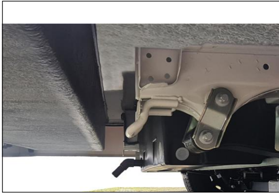
Image 4 (ex.): fin du châssis rallongé du camping-car
